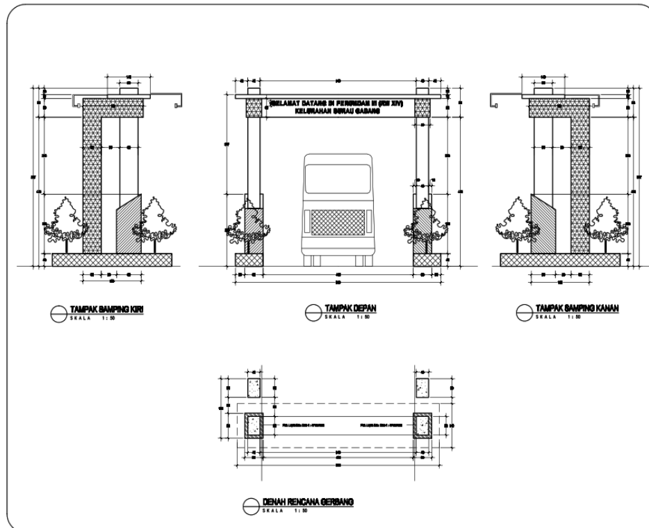
Gambar 1 Desain Gapura Pintu Masuk Di Jalan Handayani RW 14 Kota Padang
